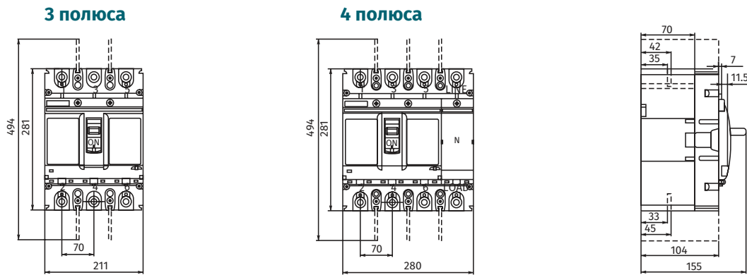
Размеры установки на щите 3 полюса
